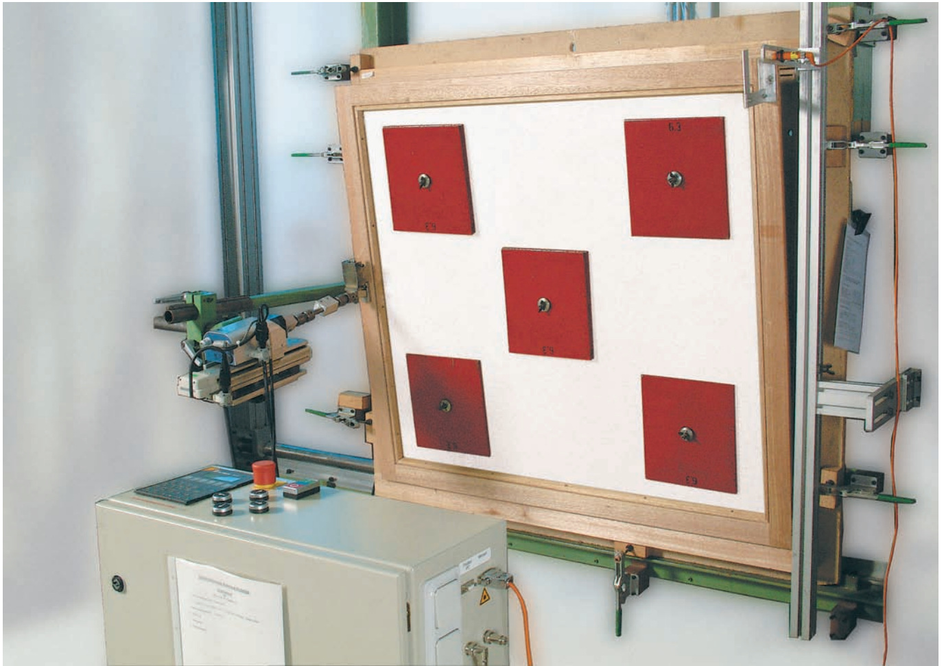
Gesamtansicht Prüfstand Drehkippschläge
